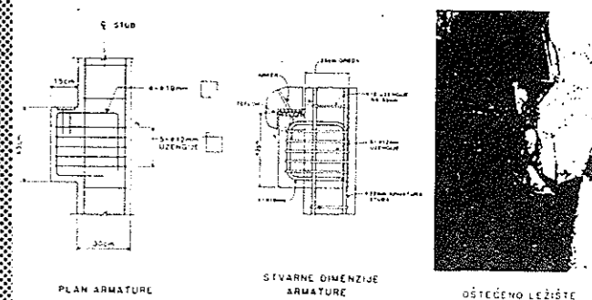
SLIKA 2 — DETALJ KRATKE BETONSKE KONZOLE — LEŽIŠTA
