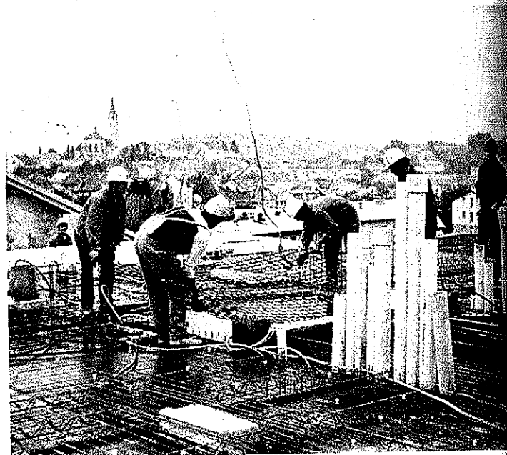
Med armaturnimi mrežami na vrhu tunnelskega opaža so položeni tudi električni kabli bodočih instalacij in pripravljene vse odprtine za prezračevalne cevi, dimnike in drugo
