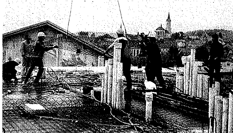
Železokrivci polagajo na vrhni del tunelskega opaža Outinord armaturo
