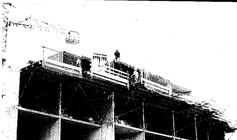
Gradnja stanovanj po sistemu Outinord se odvija zelo hitro: velik stanovanjski blok je v 4 mesecih od začetka del vseljiv
